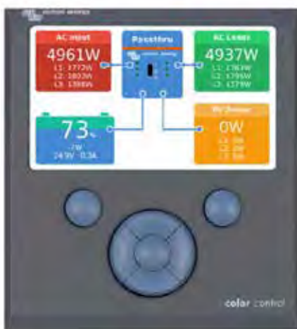
Panel Color Control con una aplicación FV
