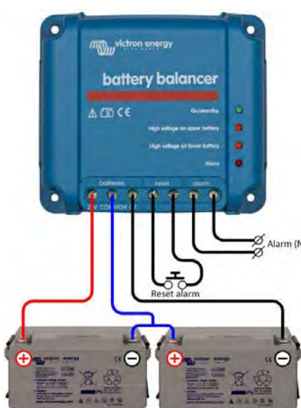
Battery Balancer conectado a dos baterías de 12V conectadas en serie (sistema de 24V)
